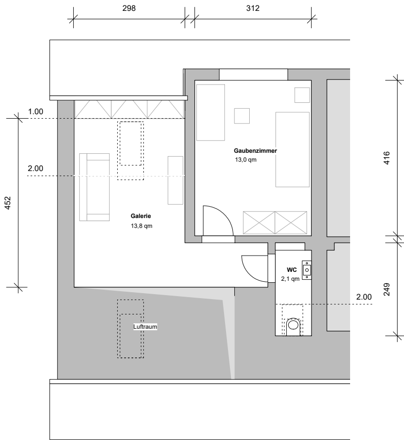
Grundriss DG
