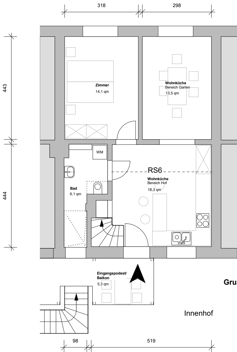
100 518 Grundriss DG
